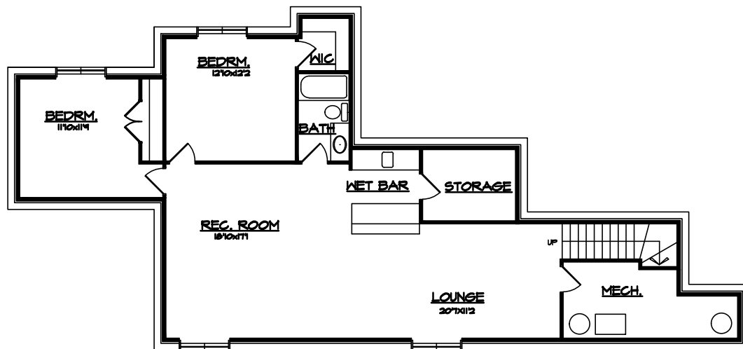
BASEMENT- 1327 S.F.
